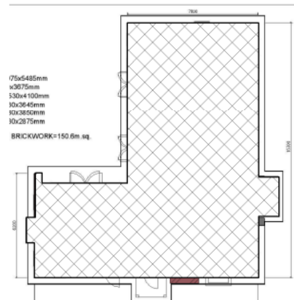
3 ORIENTATION PLAN 2 1 : 200
