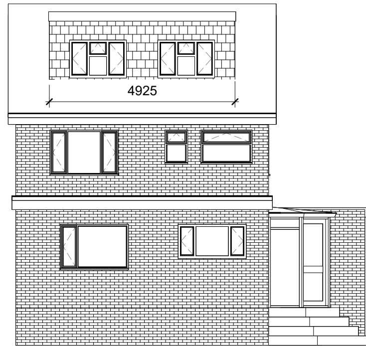
5 West 1 : 100
