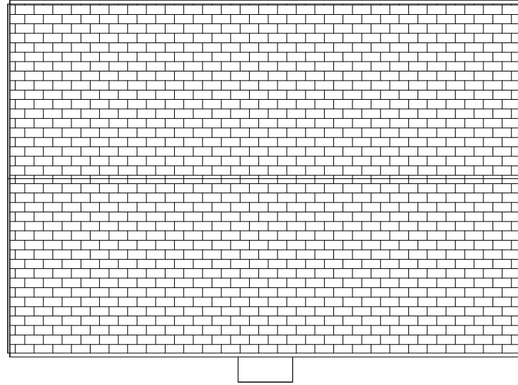
Roof Plan 1 : 100
