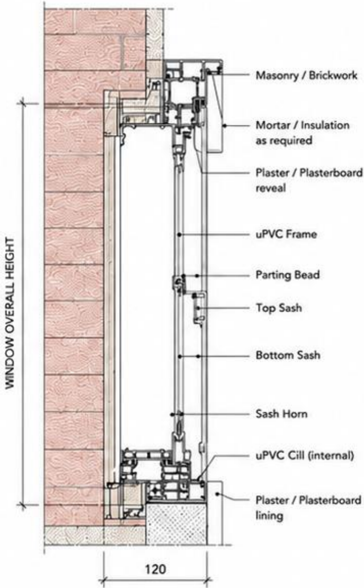
02 JAMB SECTION SCALE 1:10
