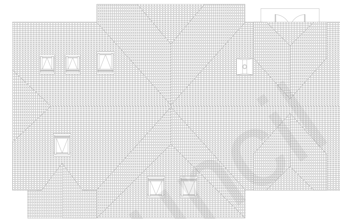
3 ROOF 1 : 100
