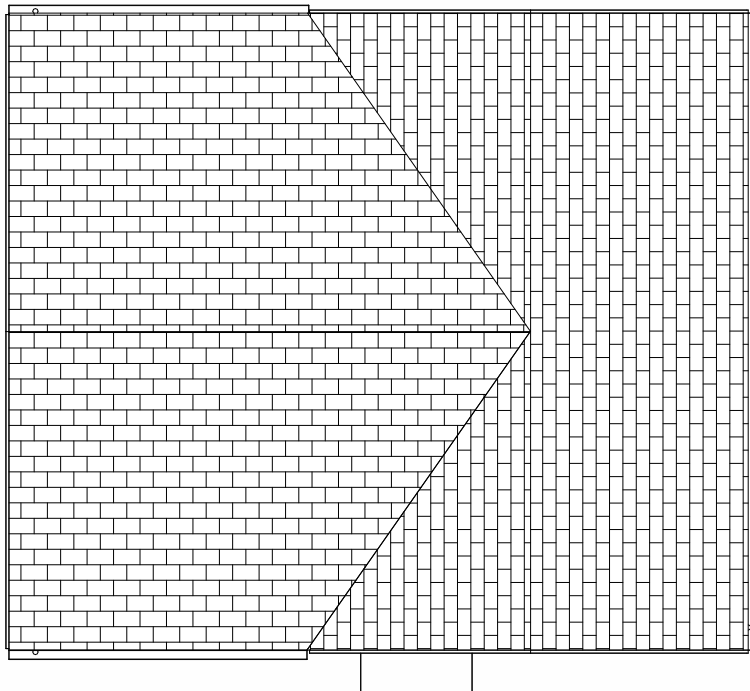
Roof Plan 1 : 100
