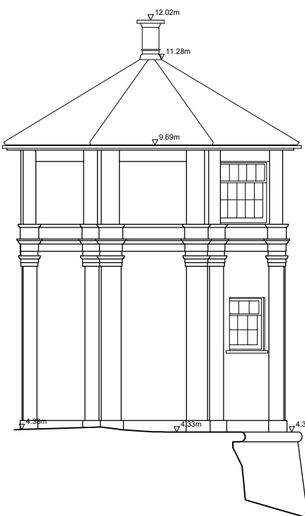
Right flank elevation
