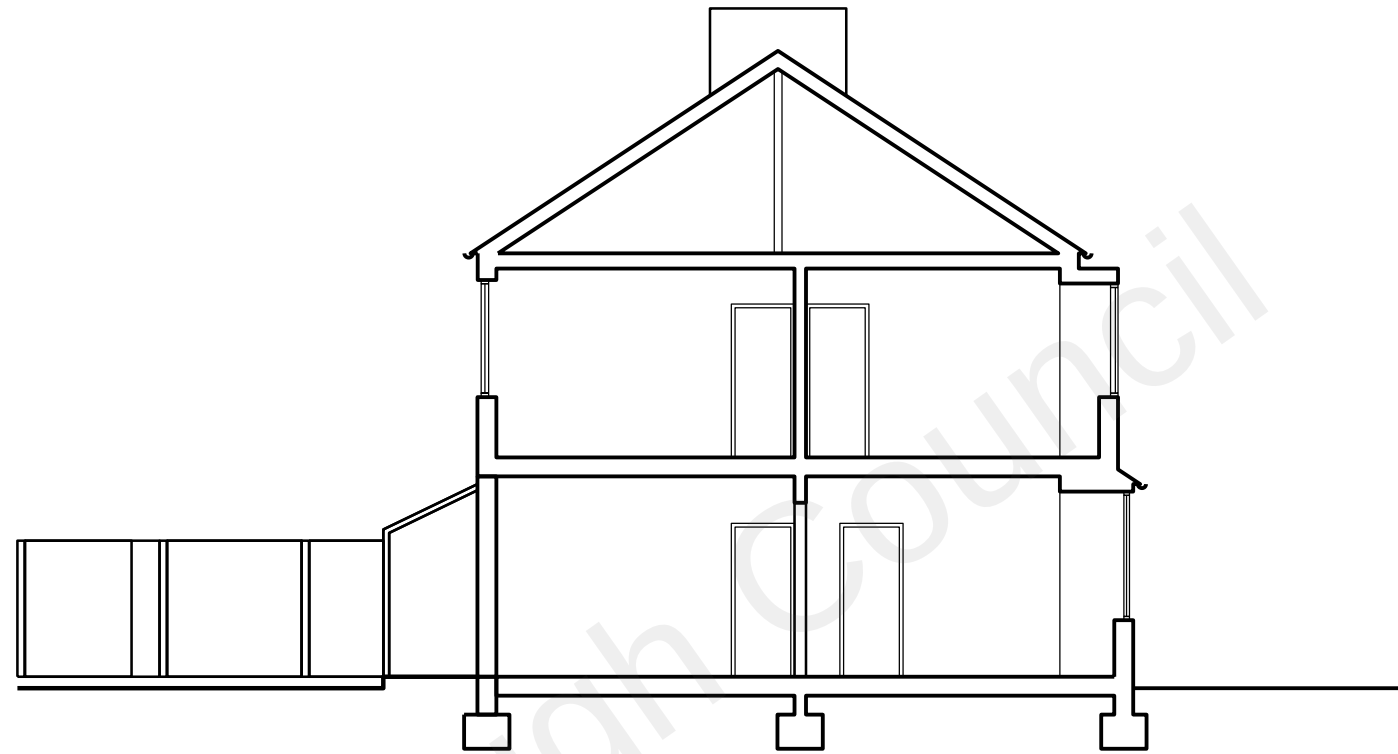
02 Section 1:100
