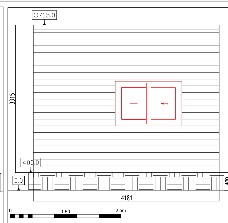
Right Elevation (D:D)
