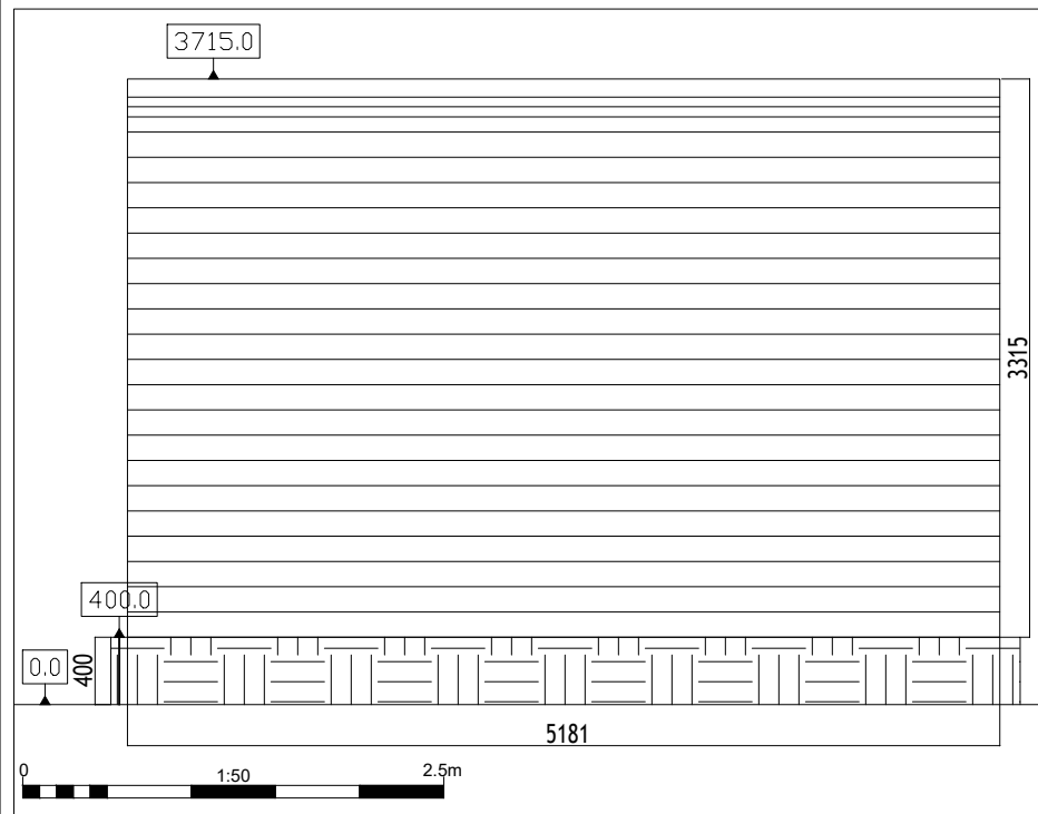
Back Elevation (A:A)
