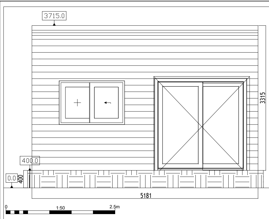
Front Elevation (A:A)
