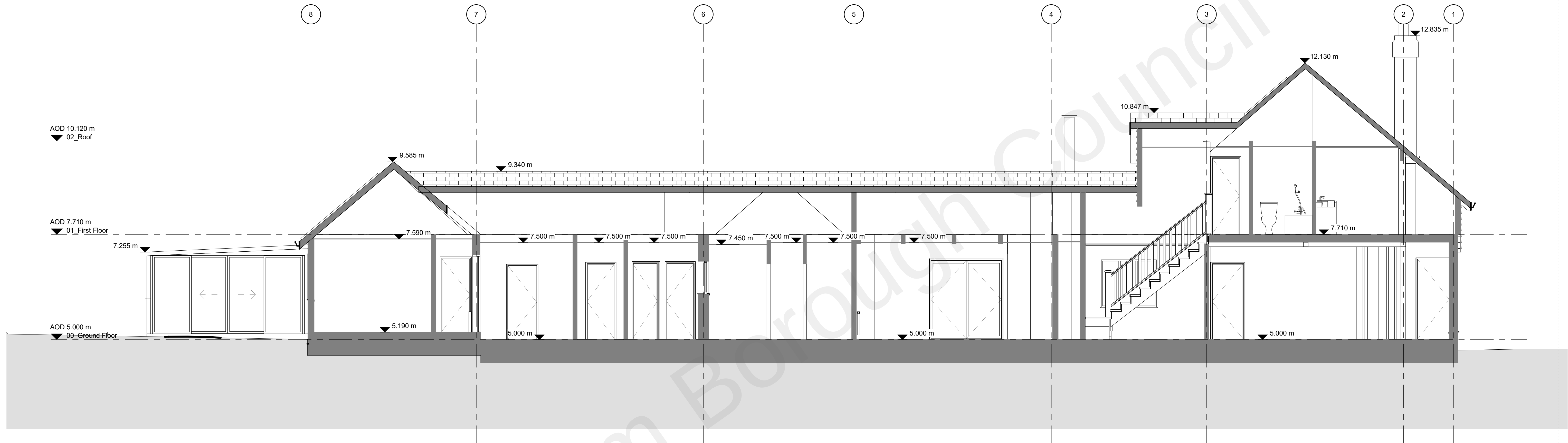
1 Existing Section A - A 1 : 50
