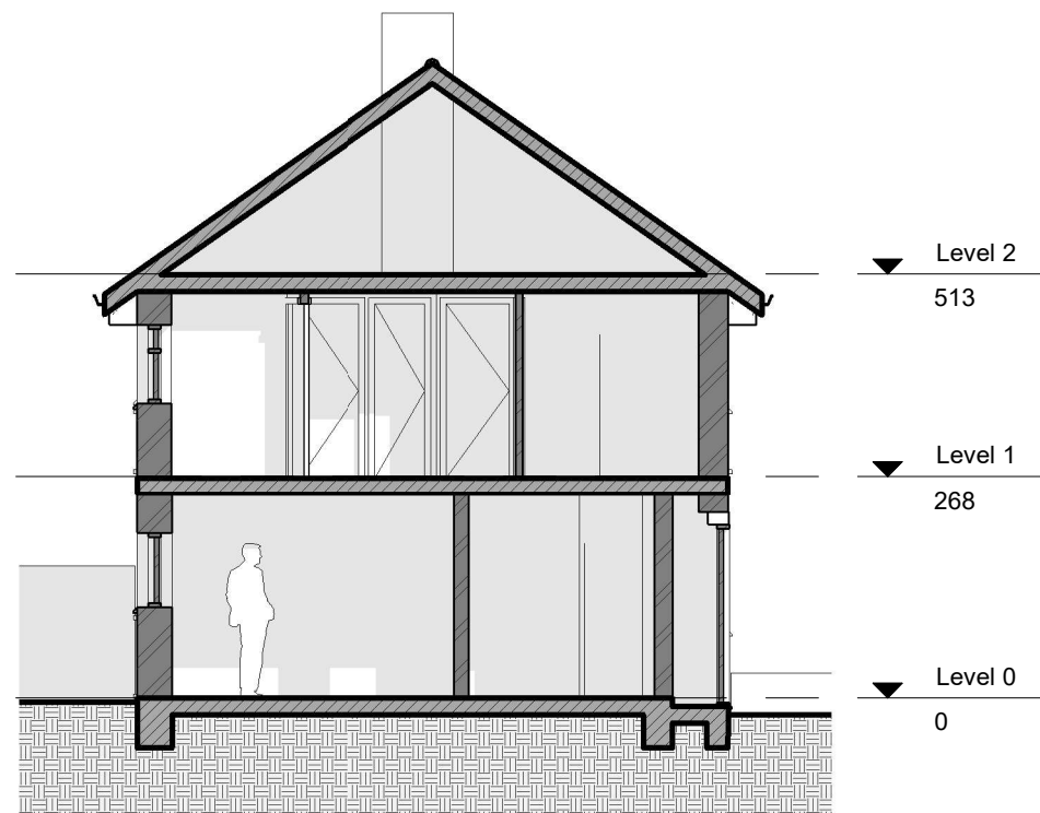
Existing Longitudinal Section 1:100
