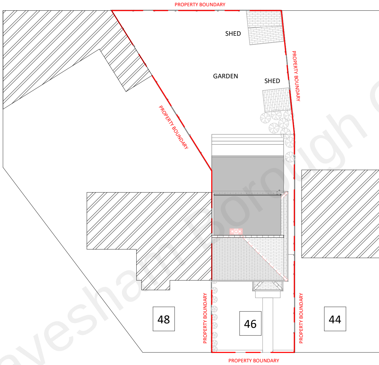
1 Site 1 : 200
