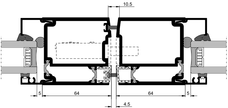
Double Door (Meeting Stile)
