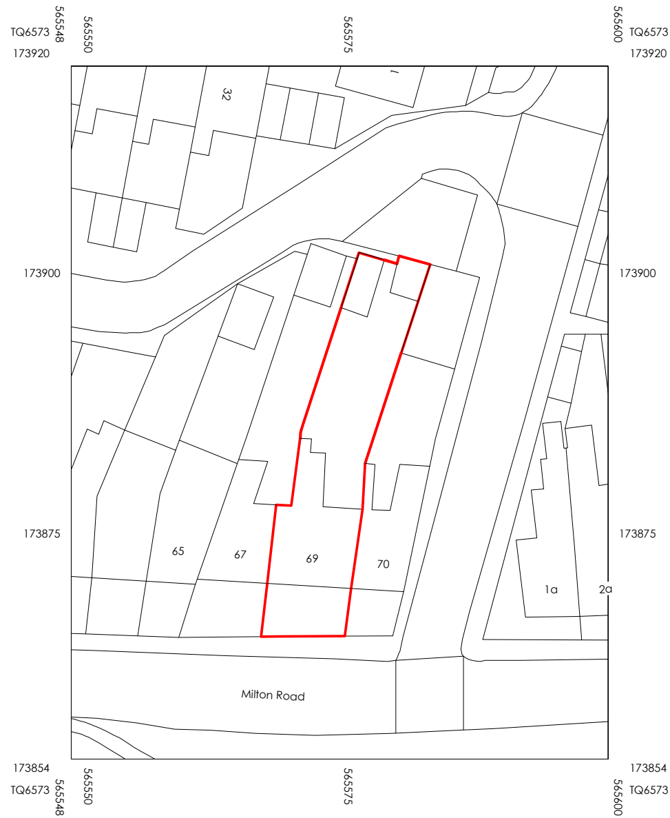
Site Plan 1 : 500
