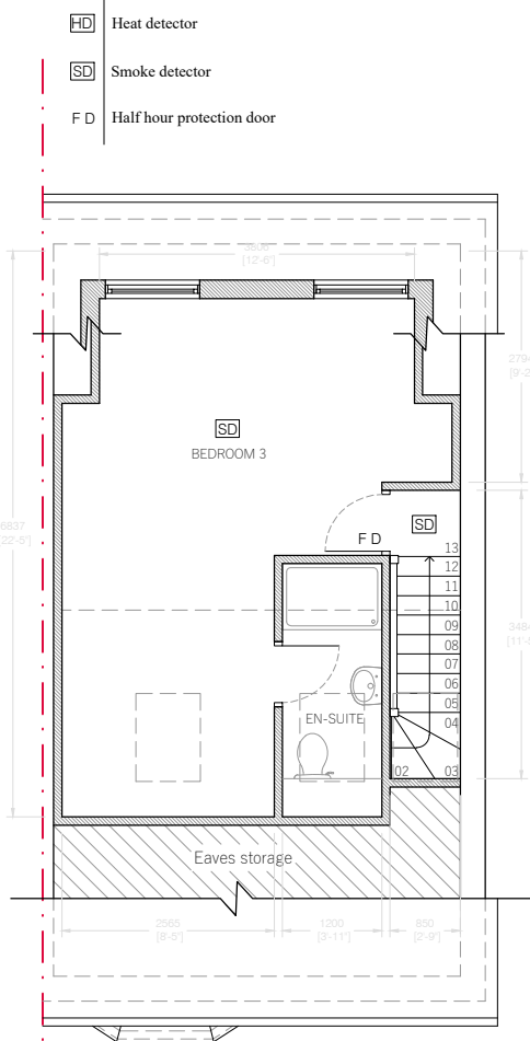
LOFT PLAN
