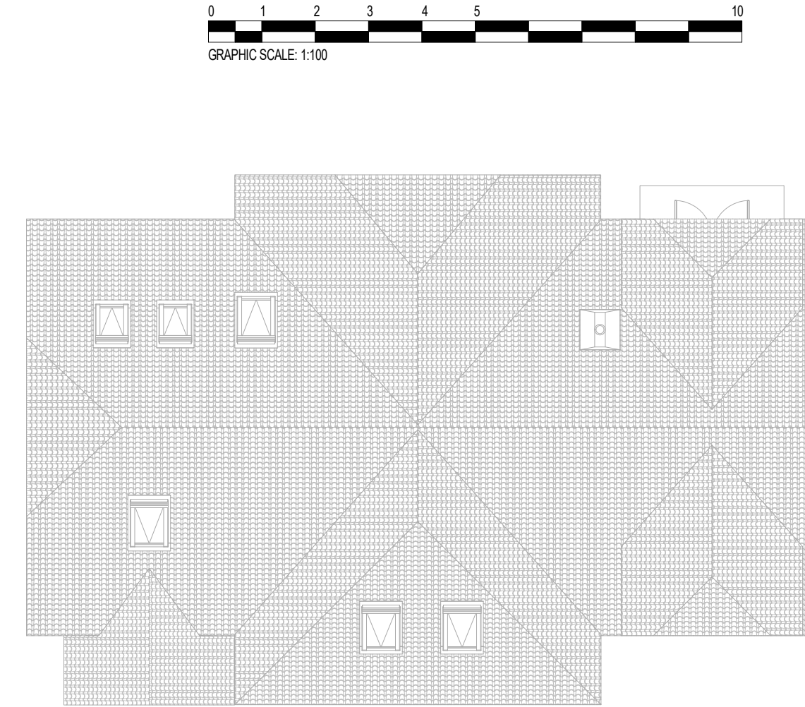
3 ROOF 1 : 100
