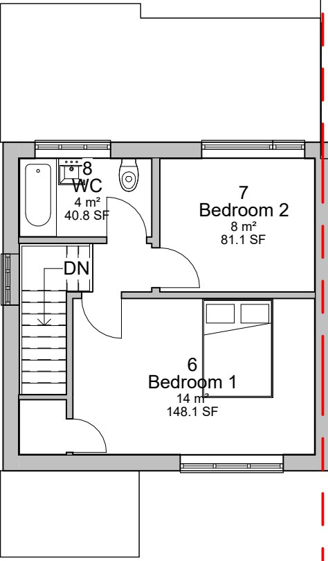
FF - Existing 1 : 100
