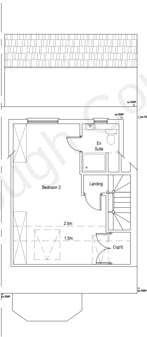
Loft Plan
