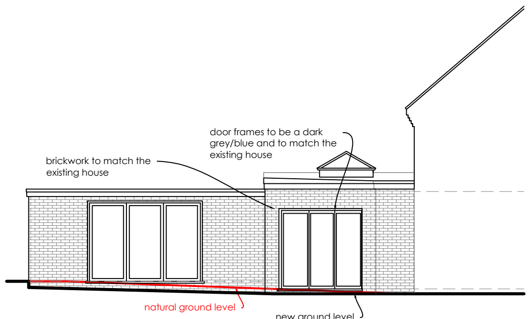
Flank elevation
