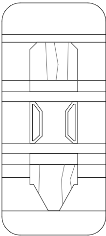
Astragal Bar Detail 1:1 @ A3
