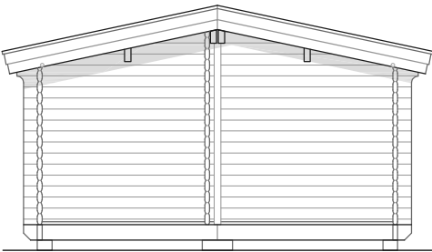
End Elevation
