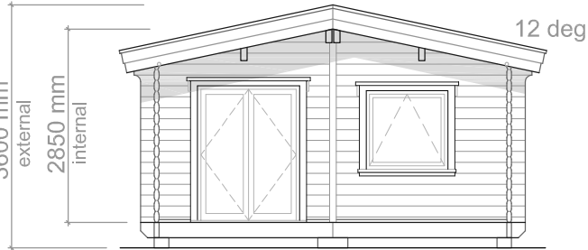
End Elevation
