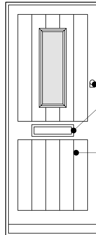
Existing Door 1:20
