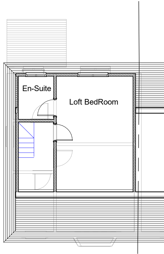
2 Ex Second Fl 1 : 100
