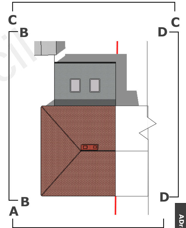
ELEVATION KEY
