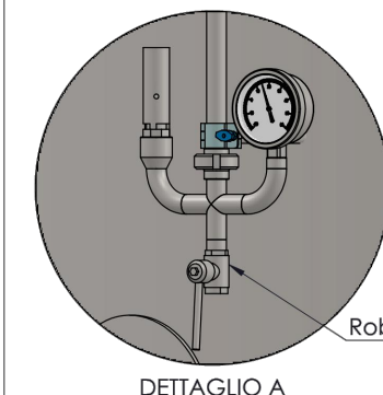
DETTAGLIO A
