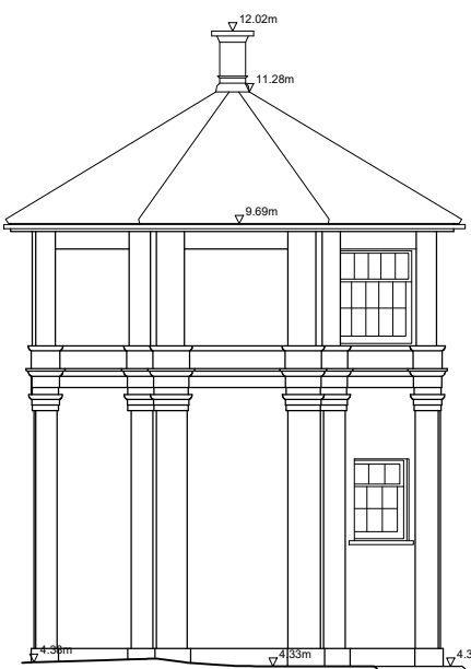
Right flank elevation
