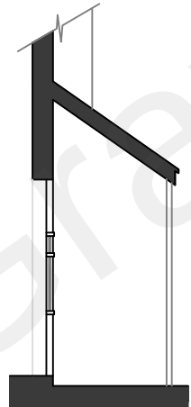
Original Section A-A 1:100
