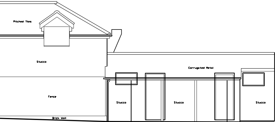
ELEVATION 1
