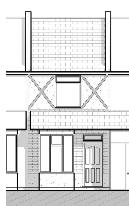
East 1 : 100
