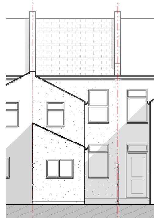
West 1 : 100
