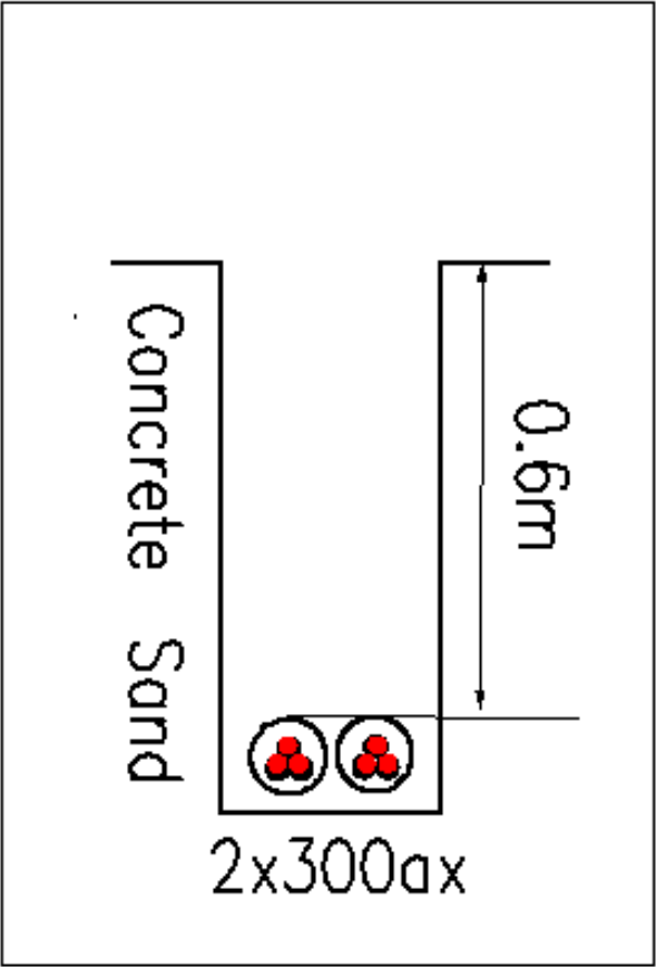
Cross Section : 2403708
