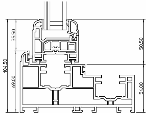
Top Jamb
