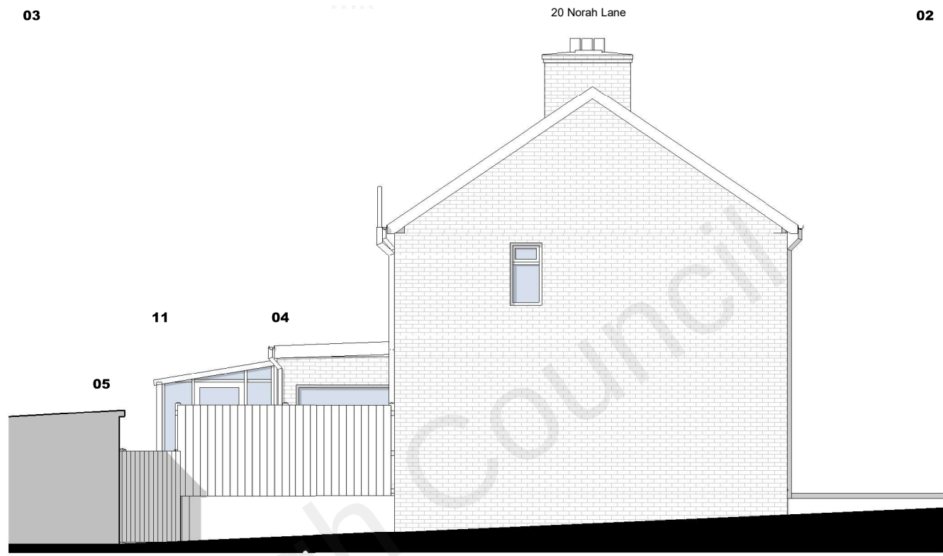
Existing Elevation 02
