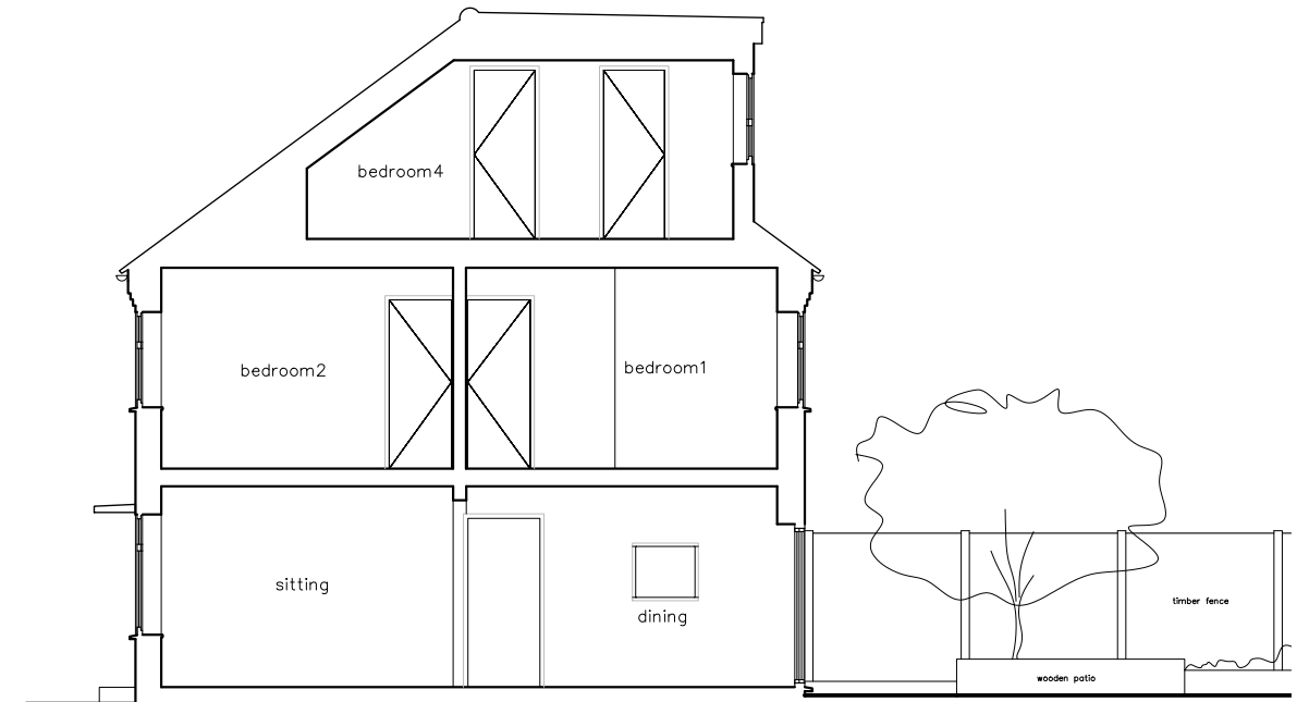
Section A-A 1:100
