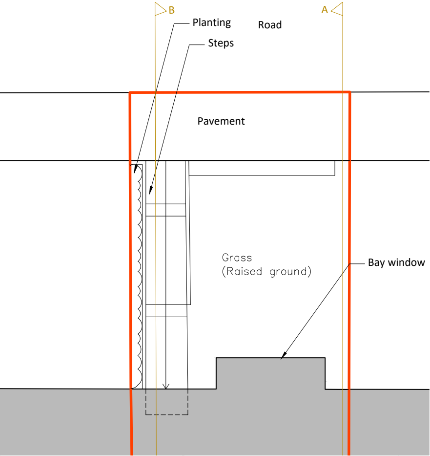
Existing Site Plan 1:100
