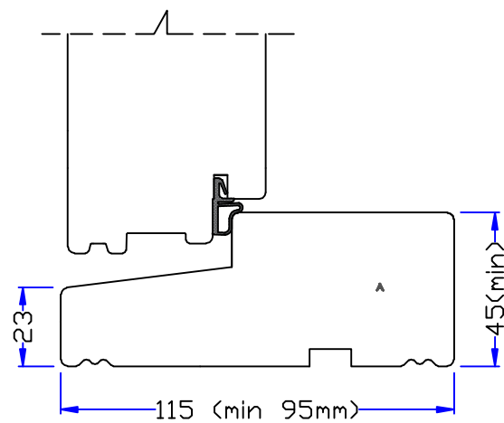
B-B Optional flush hardwood sill
