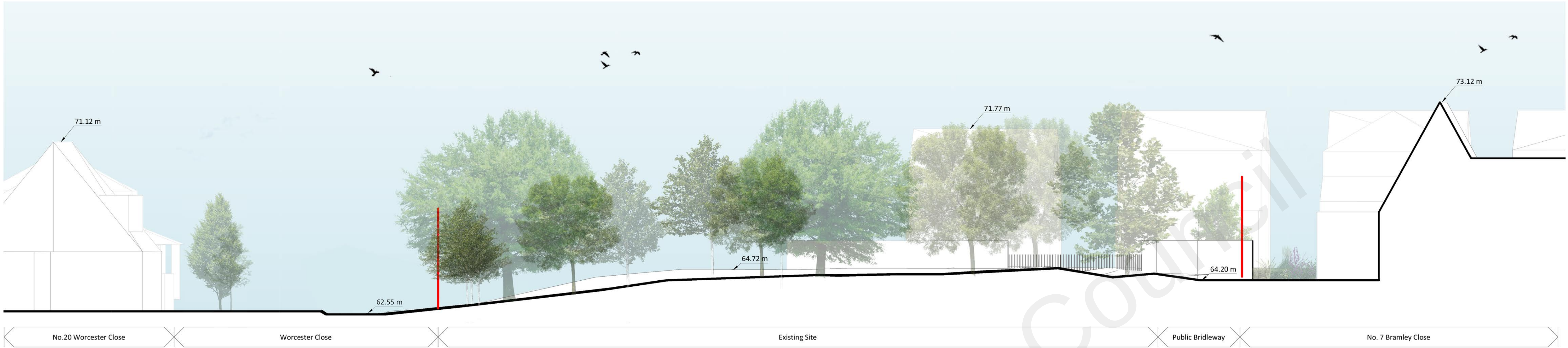
Existing Site Section AA 1 : 100
