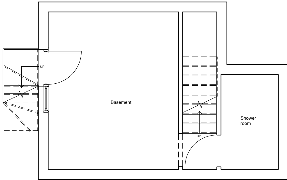
00. BF Existing 1 : 50
