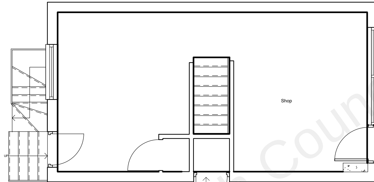
01. GF Existing 1 : 50
