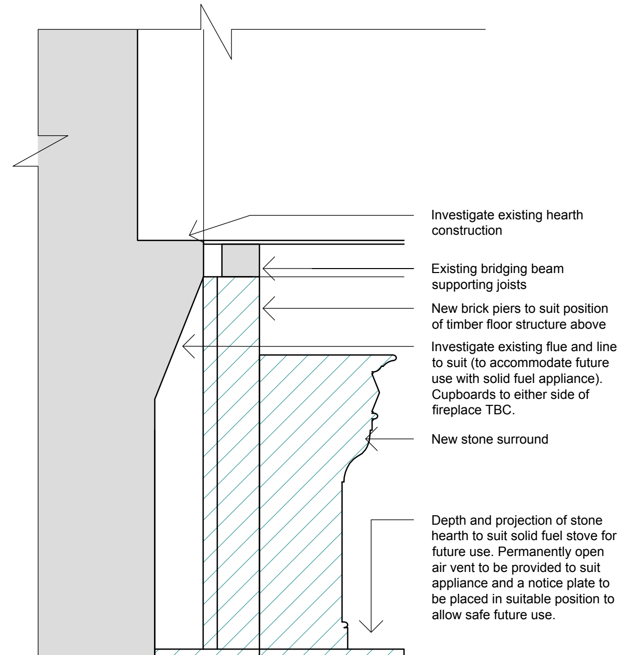
SECTION DD
