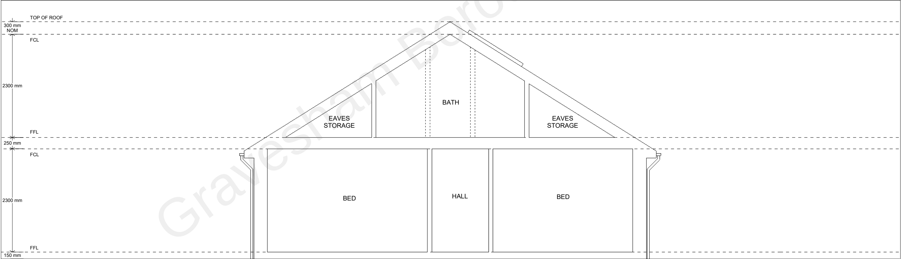
SECTION DD
