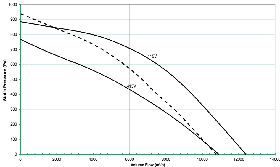
ESTOC 80-630-3 - BI101221
