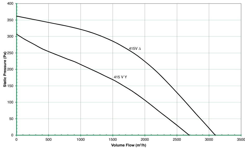
Estoc 50-355-3 - UB503544
