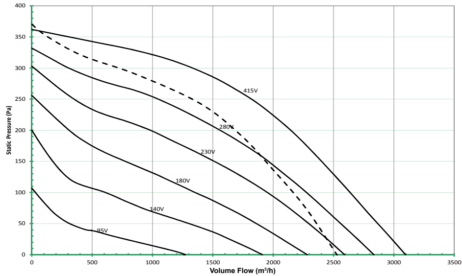
Estoc 50-355-3 - BI101216
