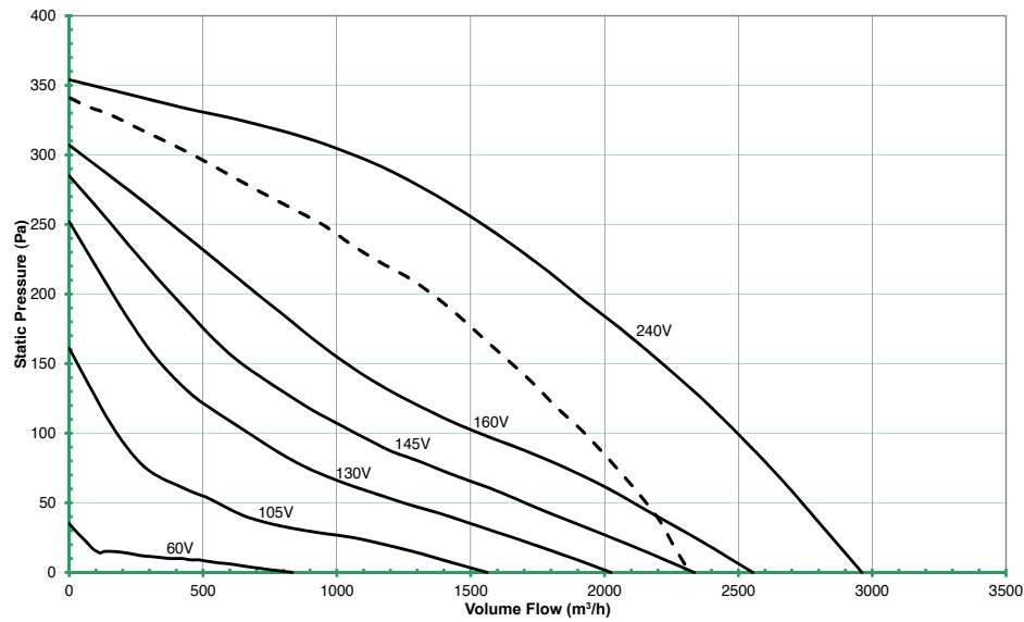
Estoc 50-355-3 - BI101216
