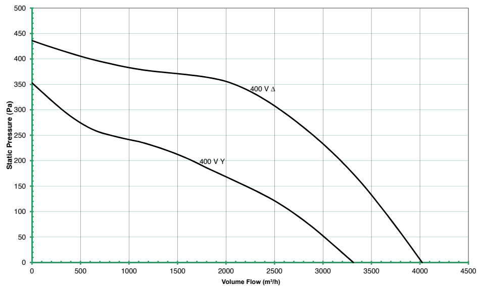
ESTOC 67-400-3 - UB674044
