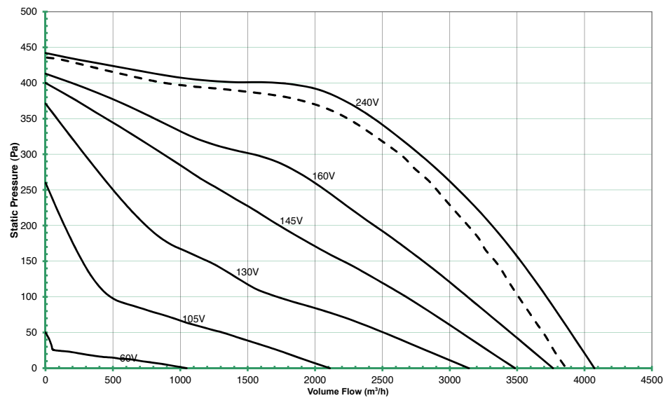
ESTOC 67-400-3 - BI101217
