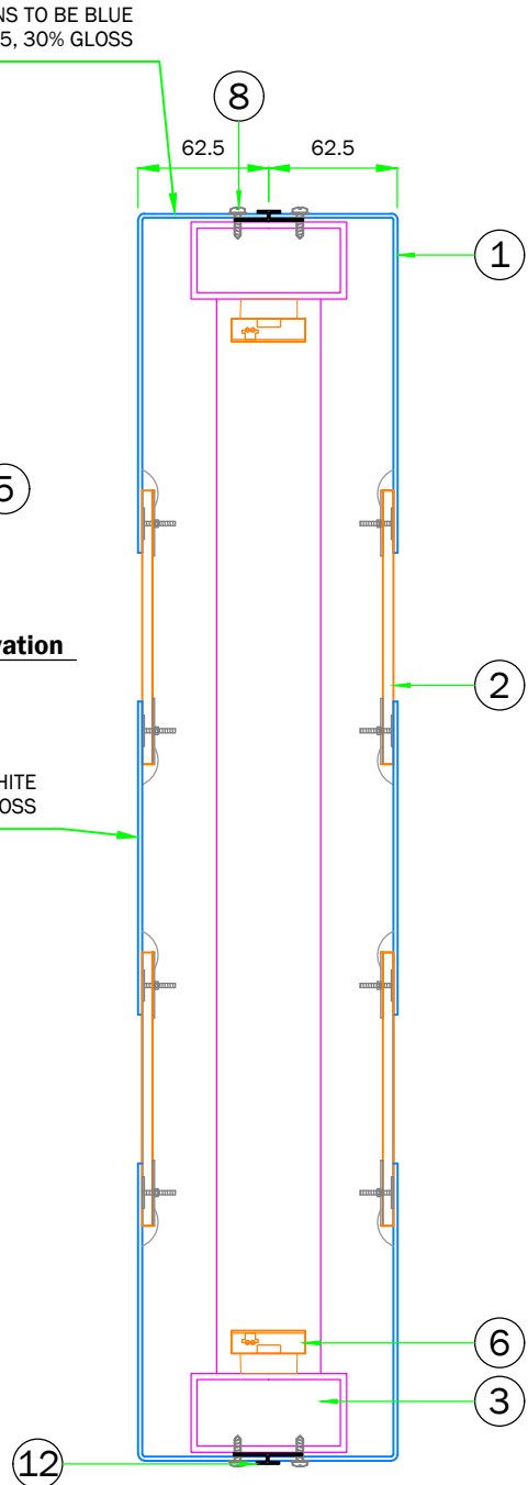
Section A-A scale 1:4
