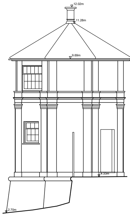
Left flank elevation
