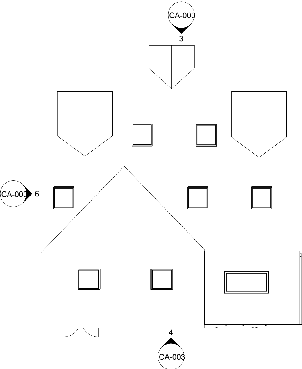
2 Roof Plan 1 : 100
